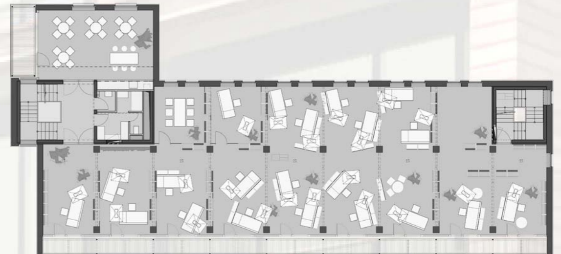
Grundriss 1.OG
